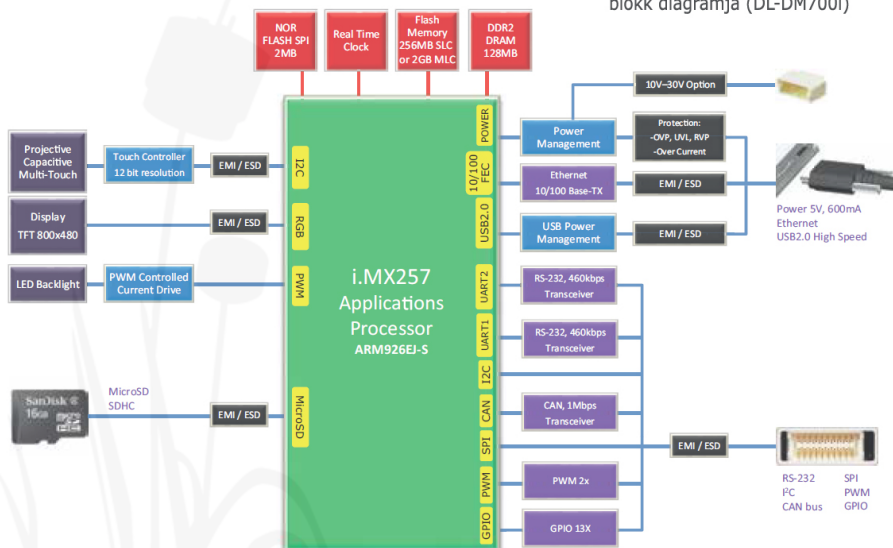
Smart Display Modul „i” sorozat blokk diagramja (DL-DM700i)
